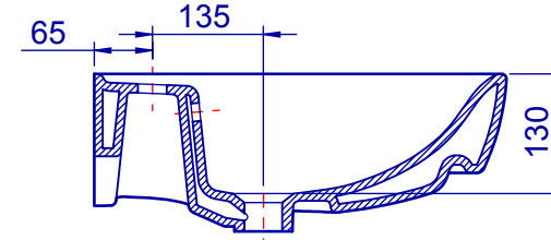
A-A KESİTİ
