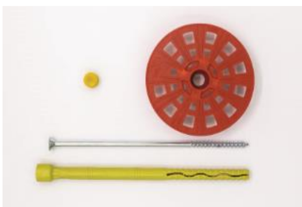
Flansa+tija filetata+cilindru expandare + capacel
