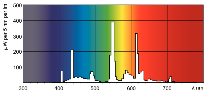
Culoare lumina /840
