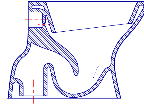
A-A KESİTİ
