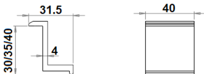
Fig. 1 - Dimensiuni clema de capat
