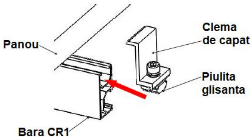
Fig. 2 - Instalare panou fotovoltaic - clema de capat
