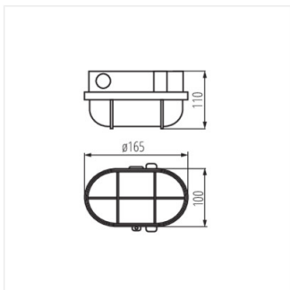
MILO 7040T
