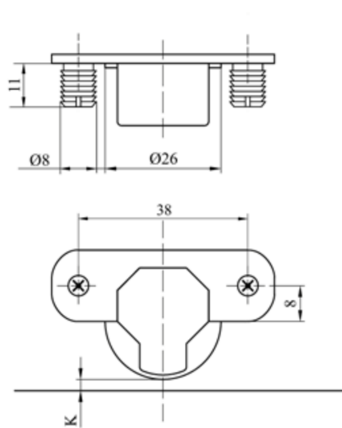
Prindere cu dibluri
