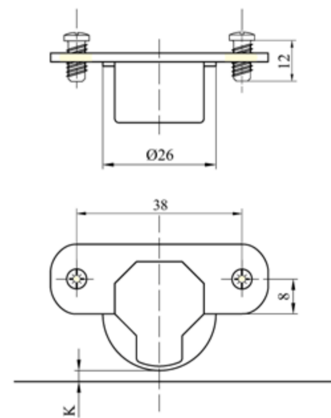
Prindere cu euroșuruburi
