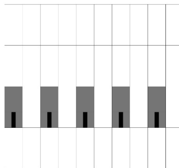
Intre 30° - 45° fiecare a 2-a tigla parazapada
