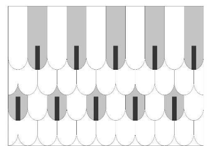
Peste 45° - 6 buc/ml fiecare in tabla de sah
