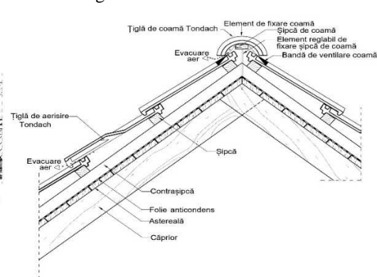
Fig.2 Secțiune zona coamei
