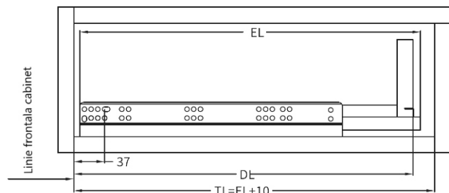
Sertare clasice
