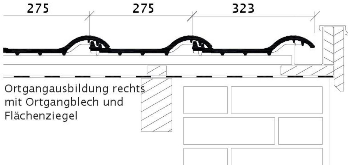
Desen tehnic produs BALANCE Țiglă laterală dreapta cu proeminența dublă OFR
