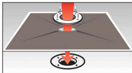
Element cu forma patrat din PVC, cu dimensiuni de 425 mm x 425 mm, pentru hidroizolarea elastica si etansarea unui sifon de scurgere
