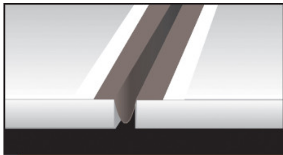
Pozitionarea Mapeband PE 120 sub forma literei omega intr-un rost de dilatare
