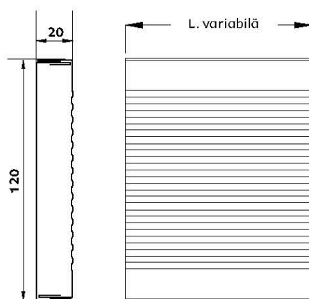
① Casetă x120
