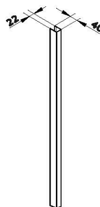
② Profil metallic de fixare pe stâlp U20
