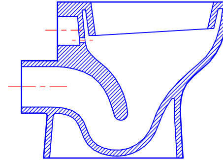
A-A KESİTİ
