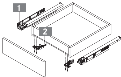
sertar cu 4 laterale
