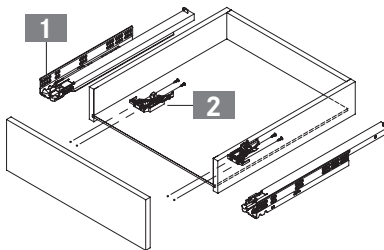
sertar cu 3 laterale
