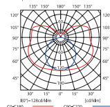
curba de difuziune a luminosității / curba de răspândire a luminii \eta = 90\%
