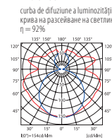
curba de difuziune a luminosității / curba de răspândire a luminii \eta = 80\%
