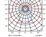
curba de difuziune a luminosității / curba de răspândire a luminii \eta = 92\%
