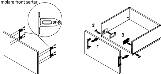
Asamblare front sertar
