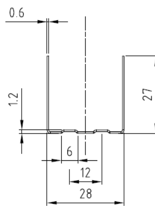
Desen tehnic UD30
