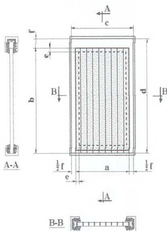
Fig. 3 - Exemple de montaj a plăcilor celulare ținând cont de dilatarea/contractia date de variațiile de temperatură
