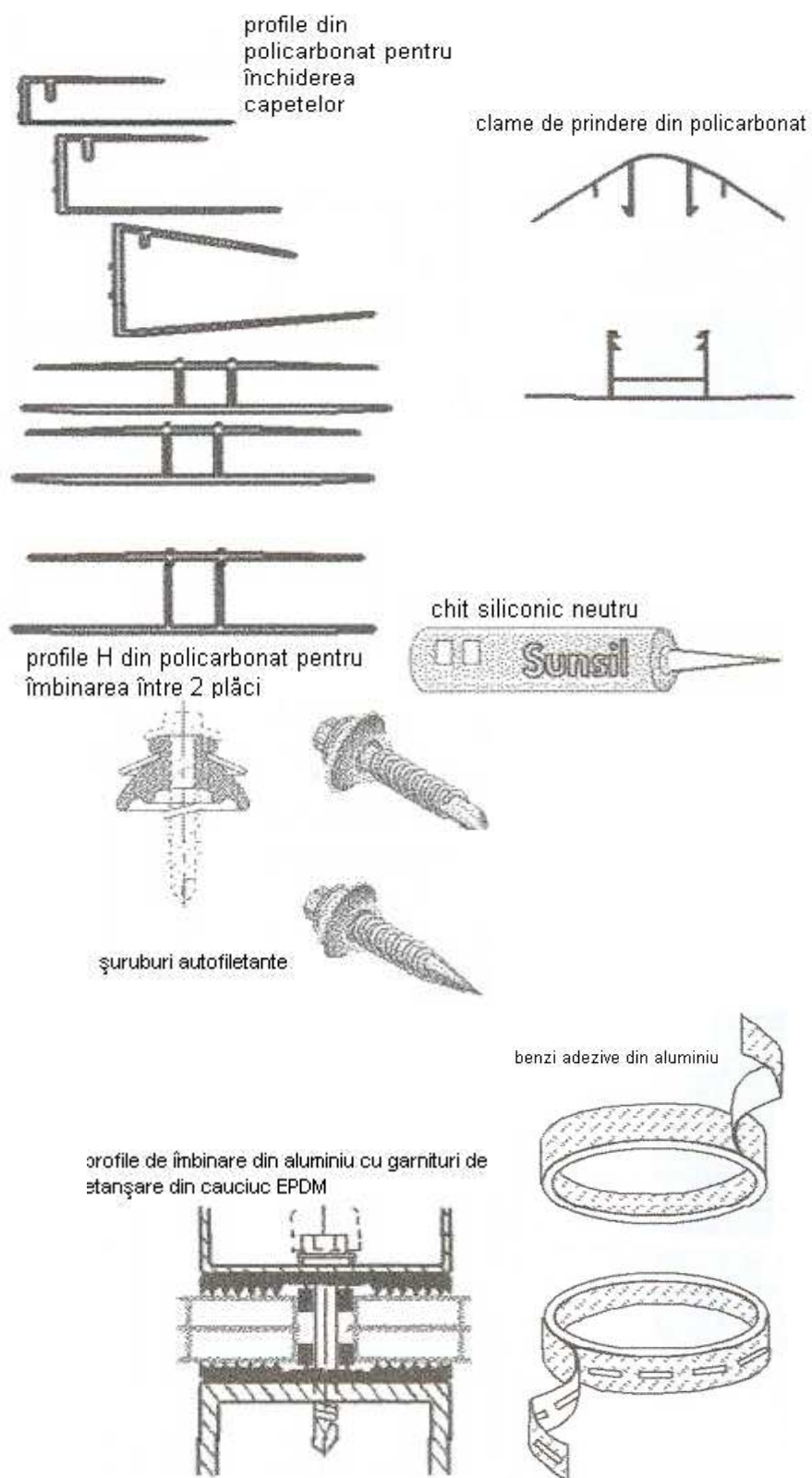
Fig.2 - Exemple accesorii de montaj a plăcilor celulare din policarbonat
