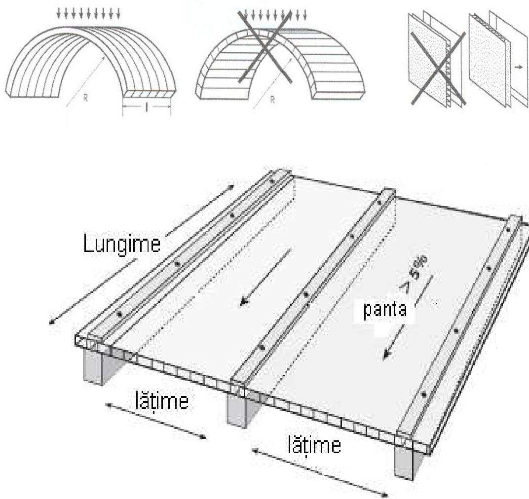
Fig. 1 - Poziționarea plăcilor celulare din polycarbonat
