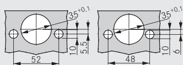
Combinatie sablon gaurire pentru Impreso
