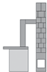
MONTAJ CORECT CU RACORD LA COS DE CARAMIDA
