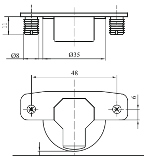
Prindere cu dibluri
