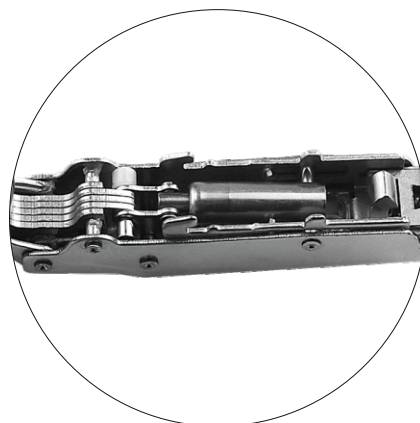
Amortizor braț balama
