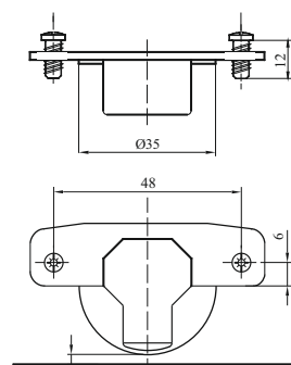
Prindere cu euroşuruburi
