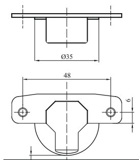
Prindere cu Holz-şuruburi
