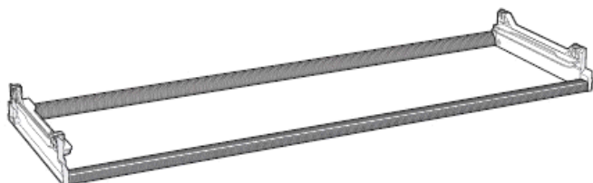
RAMĂ REGLABILĂ DIN ALUMINIU/PLASTIC PENTRU SCURGĂTOR CLASIC ȘI COMBO
