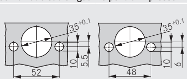
Combinatie sablon gaurire pentru Impreso
