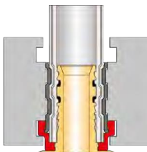
Bacul cleștelui: model "TH" - personalizat marca Tiemme Bacul cleștelui: model "TH"
