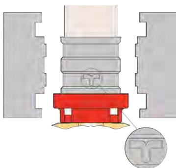
Imaginea logo-ului Imprimat pe manșon după efectuarea acțiunii de presare efectuată cu ajutorul cleștelui cu bacul model "TH" - personalizat marca Tiemme
