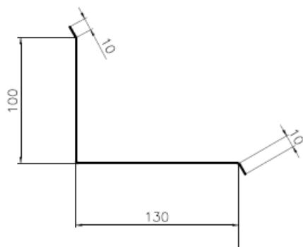
Fig.1 închidere perete mare(IP 250)
