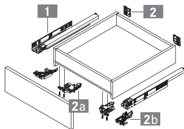
sertar cu 4 laterale
