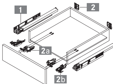
sertar cu 3 laterale
