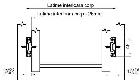
Dimensiuni (cote) instalare sertar+corp
