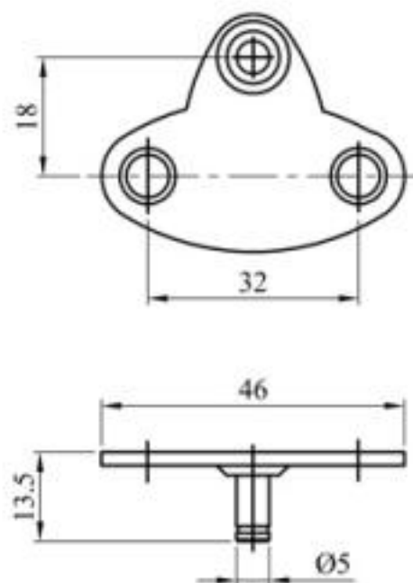
SUPPORT A Pentru fixare laterala
