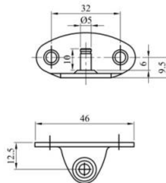
SUPPORT C Pentru usa de lemn
