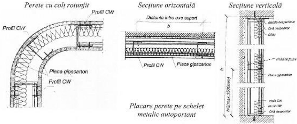
Exemplu de schelet metalic pentru perete
