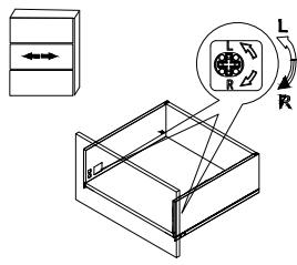
Reglaj stânga-dreapta, front sertar
