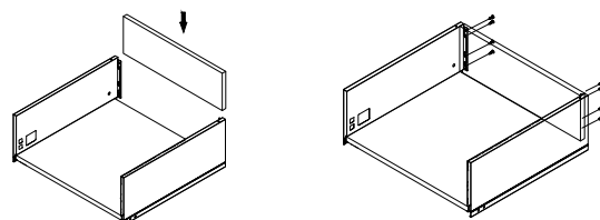
Asamblare panou spate
