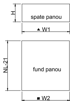
Asamblare panou fund (între cele două laterale metalice)
