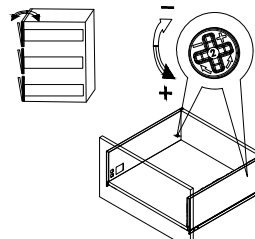
Reglaj înclinare sertar (tilt)
