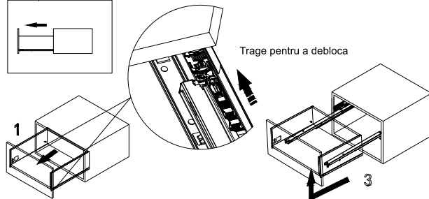
Extracție sertar
