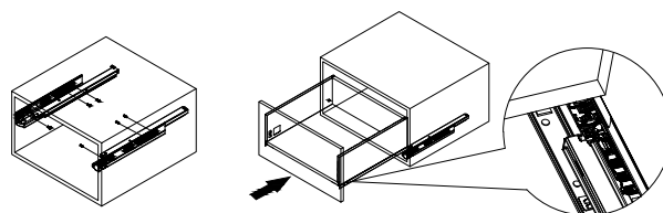
Montaj sertar pe glisieră
