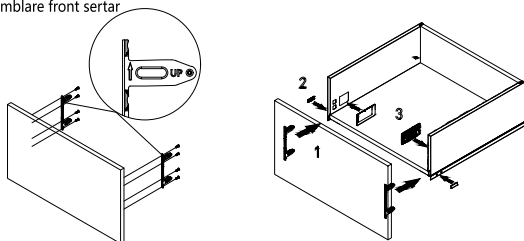
Asamblare front sertar
