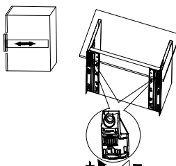
Reglaj adâncime sertar
