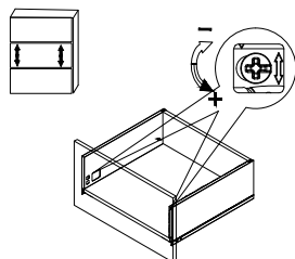
Reglaj sus-jos, front sertar
