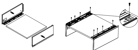
Asamblare panou fund (între cele două laterale metalice)
