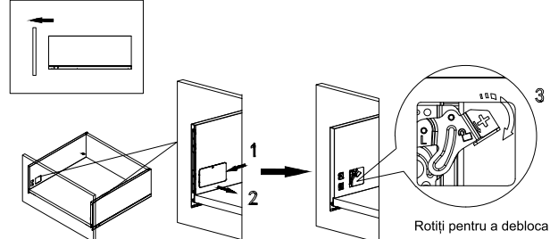
Detășare front sertar
