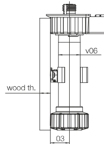
Clips metallic cu magnet pentru conectare plintă PAL de picior plastic bucătărie
