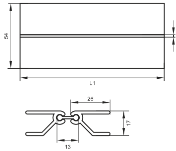
Accesoriu plintă PVC 90°
