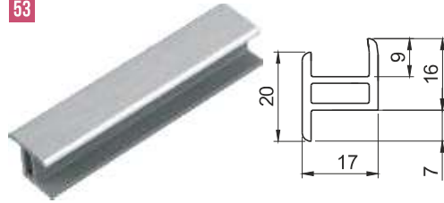
Accesorii plintă PVC, de capăt (îmbinare)
