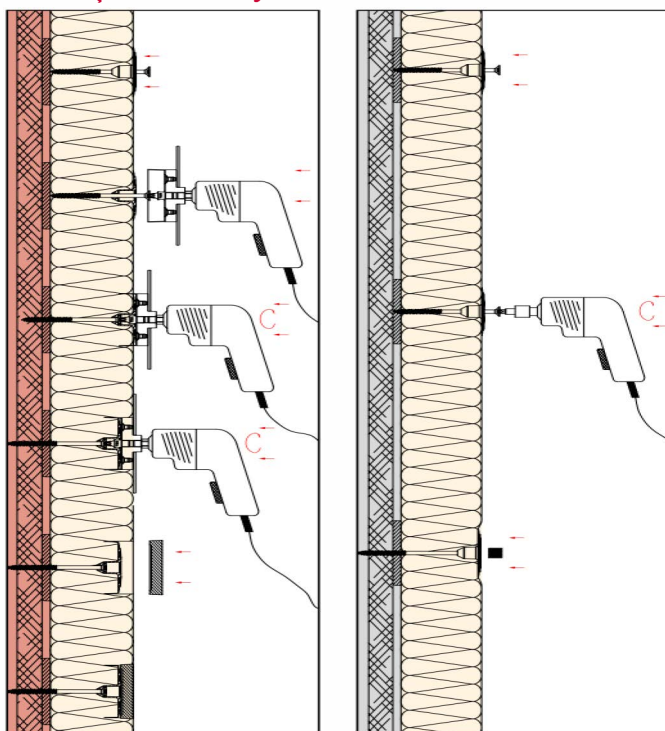
Montaj ascuns conf. principiului STR, cu rondea STR
