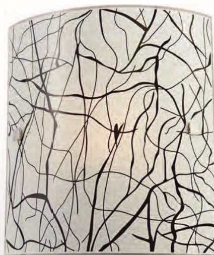
Elysia 260 KL 5813 H 26 cm L 22,5 cm W 8,5 cm 1 x E27
