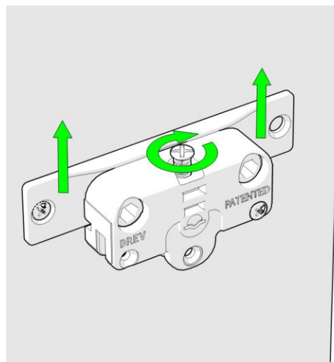
REGLARE PE VERTICALĂ FRONT
