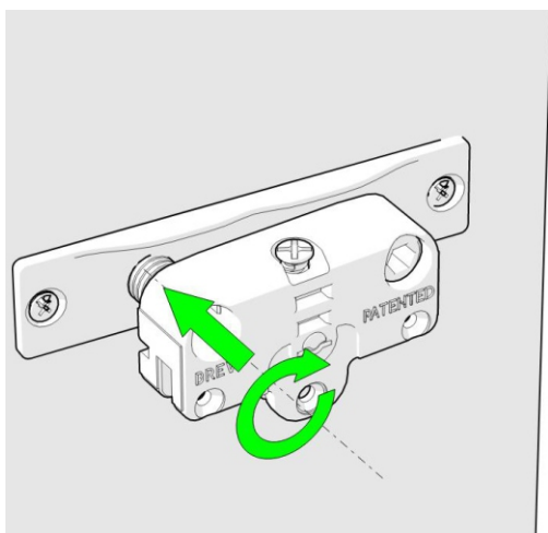
REGLARE ÎNCLINARE FRONT
