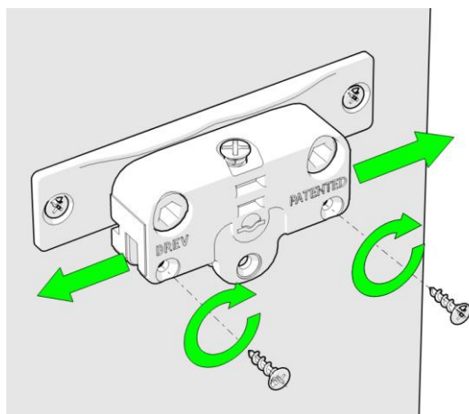
REGLARE STANGA-DREAPTA, A FRONTULUI
