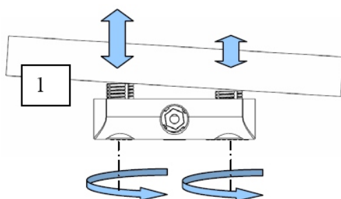
a) REGLAJ INCLINARE (1)
