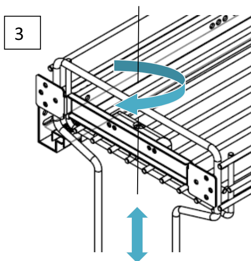
c) REGLAJ PE VERTICALĂ (3)
