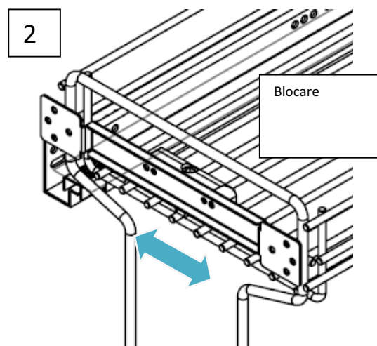
b) REGLAJ STANGA-DREAPTA (2)
