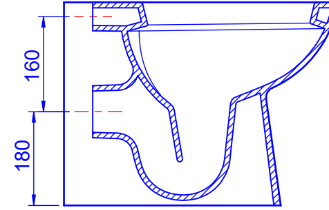
A-A' KESİTİ
