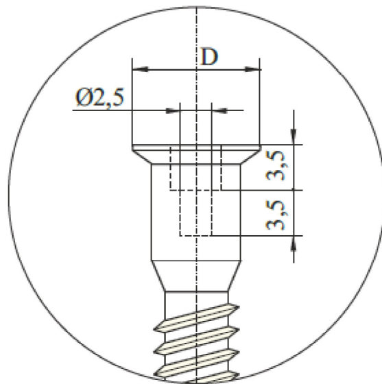
Detaliu cap șurub confirmator
