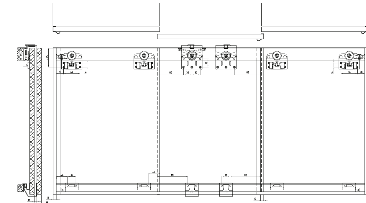
VEDERE DE SUS A AMPLASĂRII USILOR
